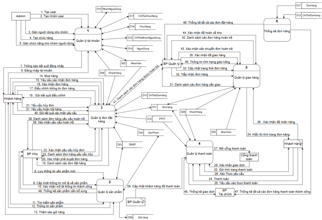
Hình 2. DFD mức 0.
